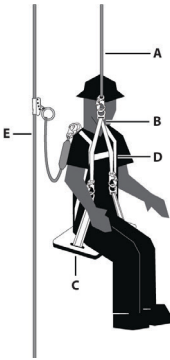
Figure 11 - Suspension et conduite par le personnel
